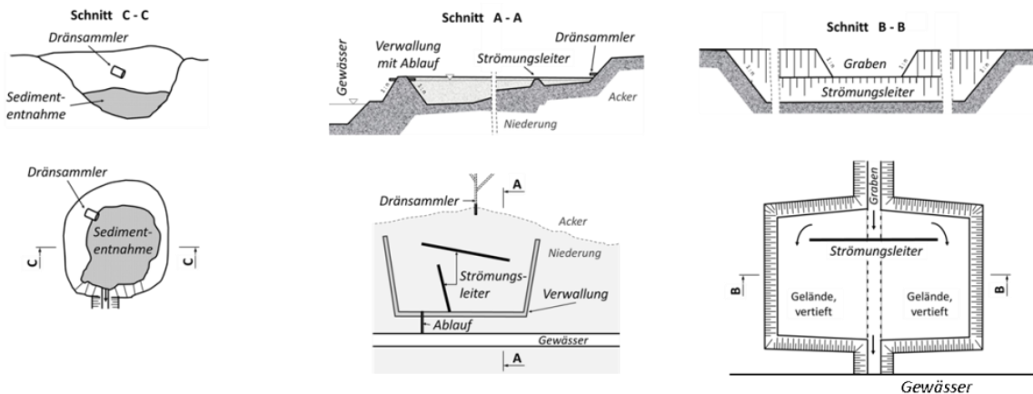
ABBILDUNG 5: GRUNDVARIANTEN DER ANORDNUNG UND GESTALTUNG EINES DRÄNTEICHES ZWISCHEN DRÄNANLAGE UND GEWÄSSER
