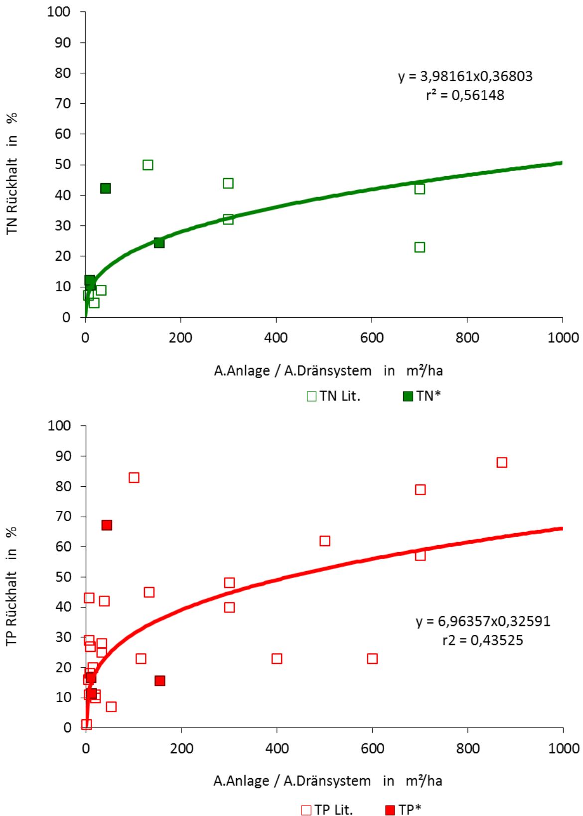
ABBILDUNG 10: GESAMTSTICKSTOFF- UND GESAMTPHOSPHOR-RÜCKHALT IN DRÄNTEICHEN ALS FUNKTION DES VERHÄLTNISSES DER FLÄCHE DES DRÄNTEICHES UND DER DRÄNFLÄCHE UNTER VERWENDUNG VON DATEN AUS DER LITERATUR UND DATEN AUS EIGENEN UNTERSUCHUNGEN (STEIDL ET AL. 2011)
