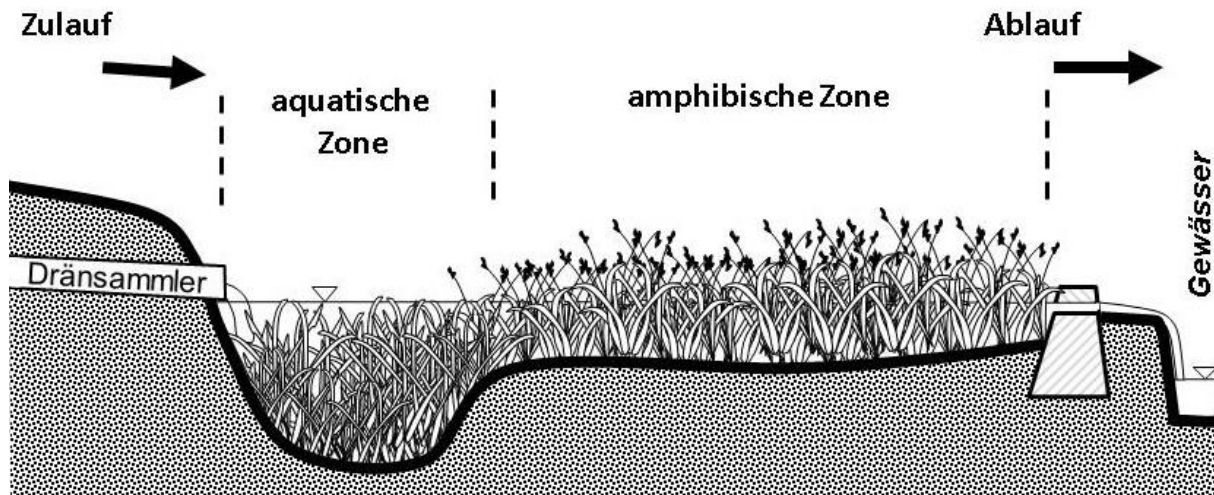
ABBILDUNG 4: LÄNGSSCHNITT DURCH EINEN DRÄNTEICH
