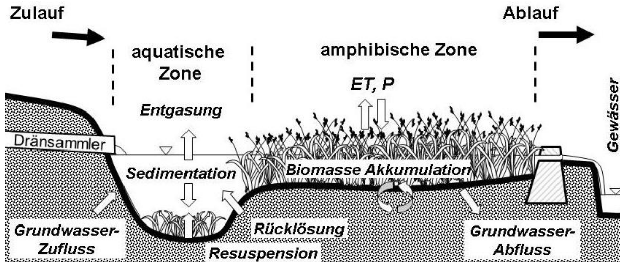
ABBILDUNG 9: PROZESSE DES RÜCKHALTS UND DER FREISETZUNG VON NÄHRSTOFFEN IN EINEM DRÄNTEICH
