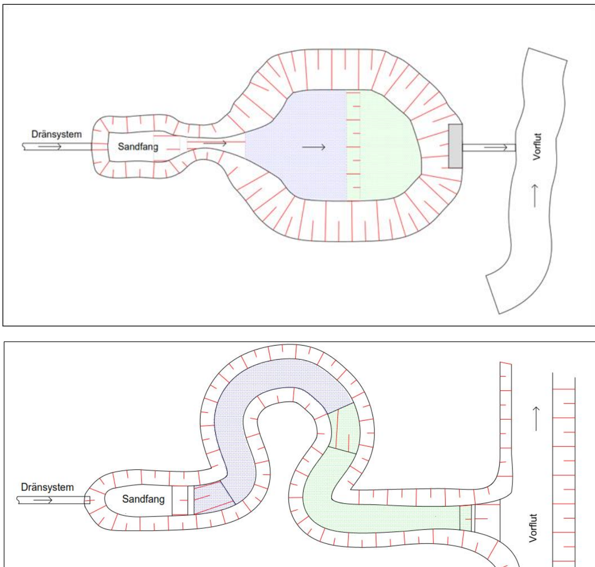
ABBILDUNG 12: SCHEMATISCHE DARSTELLUNG EINER HERKÖMMLICHEN (OBEN) UND MÄANDRIERENDEN (UNTEN) TEICHAUSFÜHRUNG MIT ZONIERUNG (BLAU = AQUATISCHE ZONE ; GRÜN = AMPHIBISCHE ZONE)
