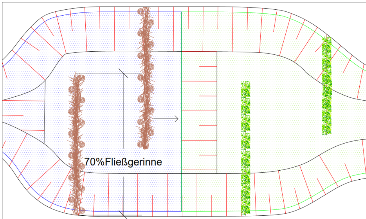
ABBILDUNG 13: PRINZIP DER FLIEßLEITSYSTEME IN DEN VERSCHIEDENEN TEICHZONEN (BRAUN = AQUATISCH; GRÜN = AMPHIBISCHE ZONE)
