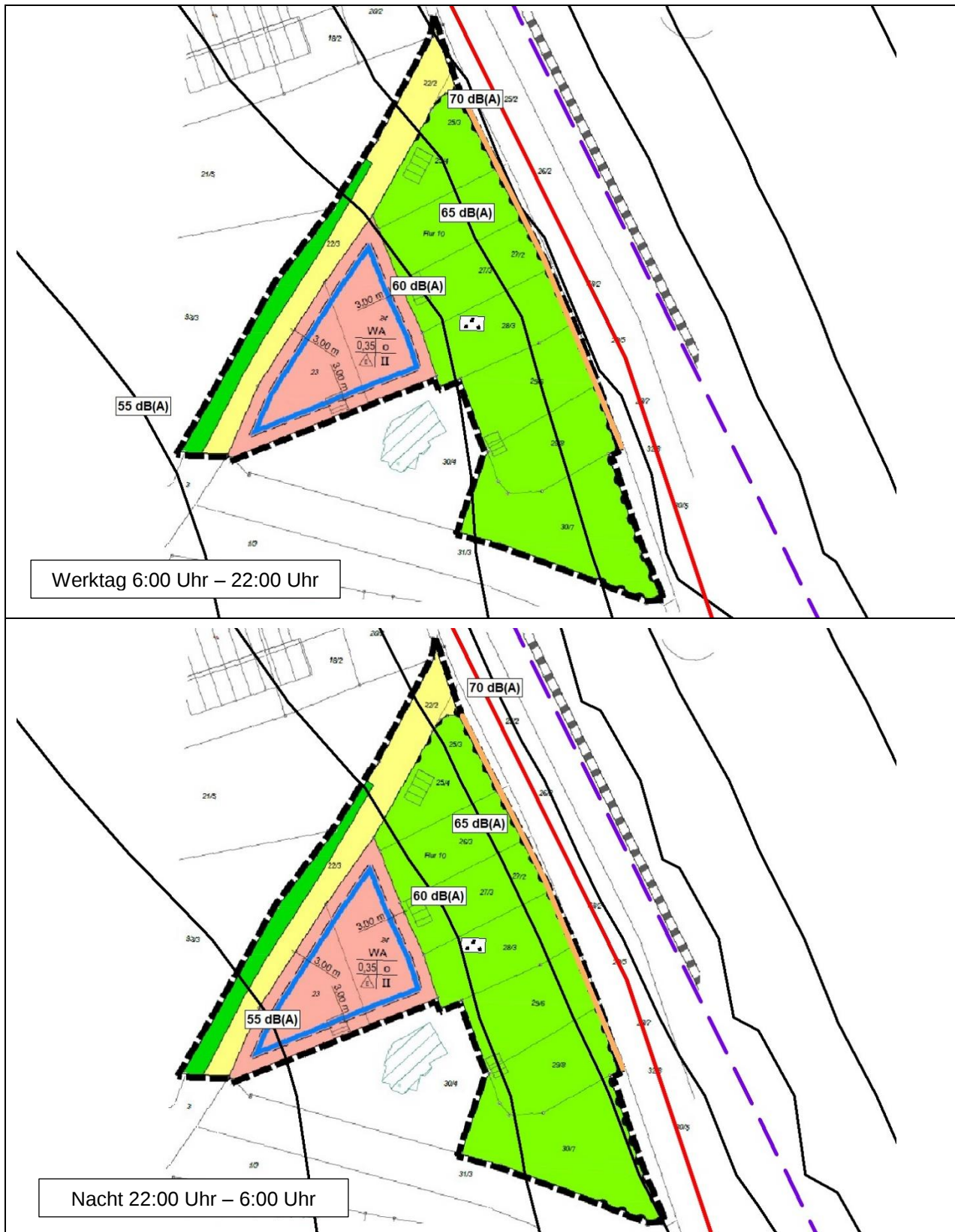
Abbildung 6: Ergebnisse der Rasterberechnung (Isolinien) – Lärmschutzwall h = 3,00 m obere Abbildung: Werktag 6:00 Uhr - 22:00 Uhr untere Abbildung: Nacht 22:00 Uhr - 6:00 Uhr
