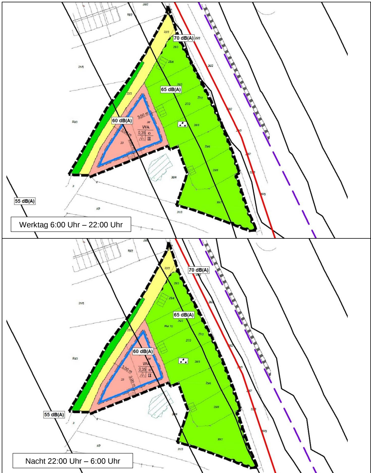
Abbildung 5: Ergebnisse der Rasterberechnung (Isolinien) - Ausgangssituation
