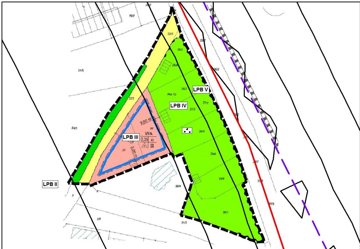
Abbildung 7: Lärmpegelbereiche unter Berücksichtigung eines Zuschlages von 3 dB(A) auf Grundlage der Ergebnisse der Rasterberechnung für die Ausgangssituation Werktag: 6:00 Uhr – 22:00 Uhr
