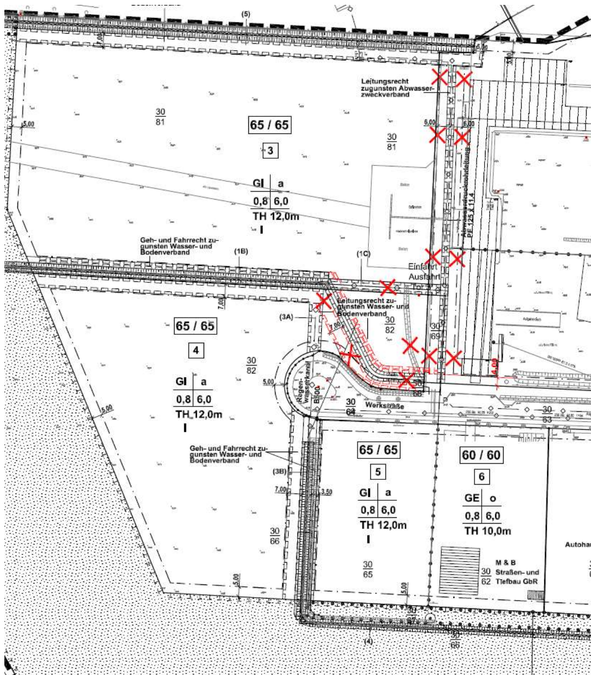
Auszug 1. Änderung des Bebauungsplanes Nr. 15/1 für das Gewerbe- und Industriegebiet „Steegener Chaussee / Holzwerke“ (Änderung Graben)
